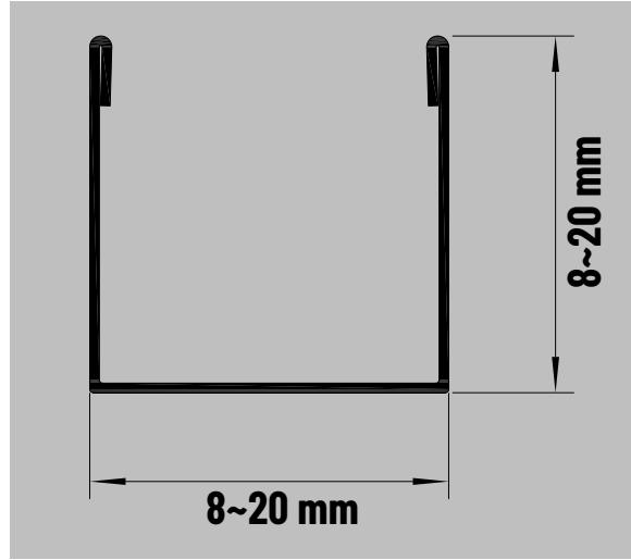
Teknik Çizim / Technical drawing
