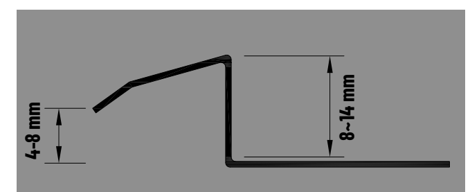
Teknik Çizim / Technical drawing
