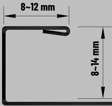
Teknik Çizim / Technical Drawing
